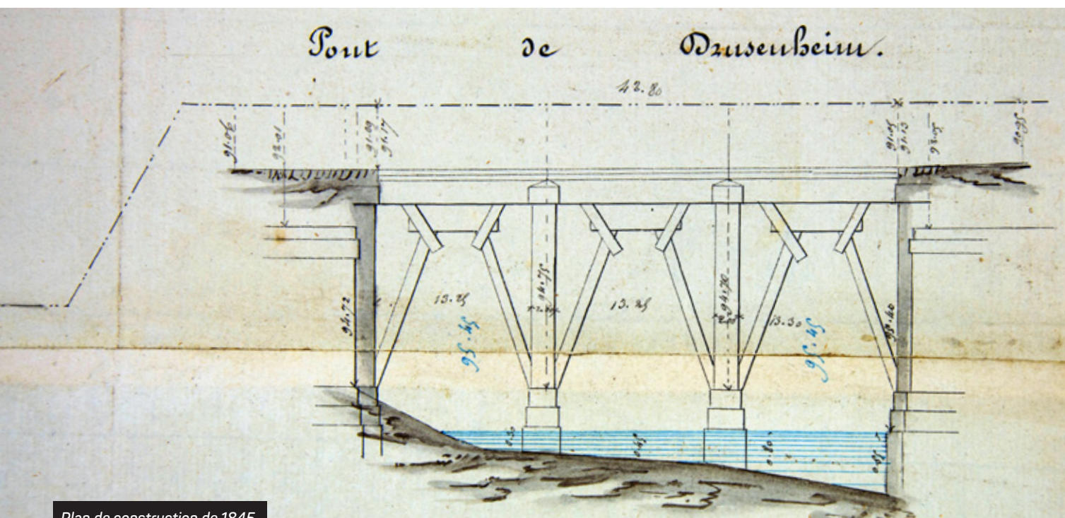
Plan de construction de 1845
